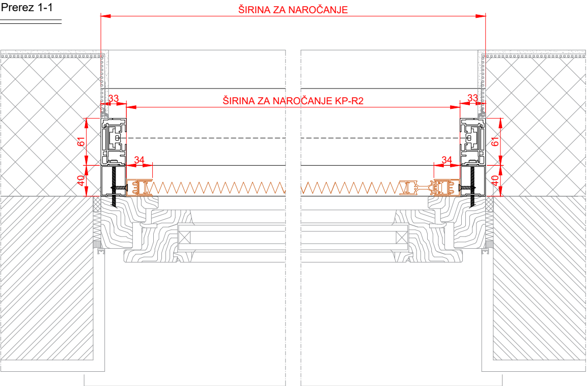
Prerez 1-1
