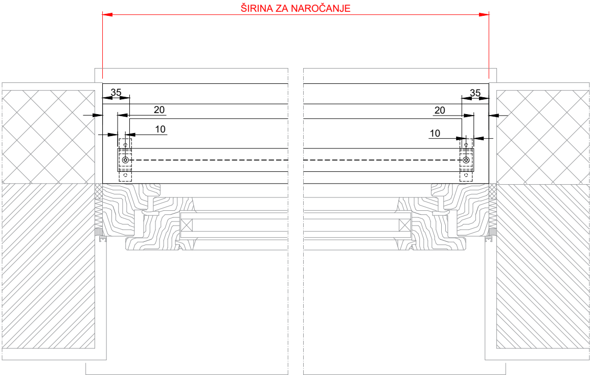
Prerez 1-1
