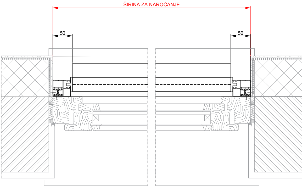
Prerez 1-1
