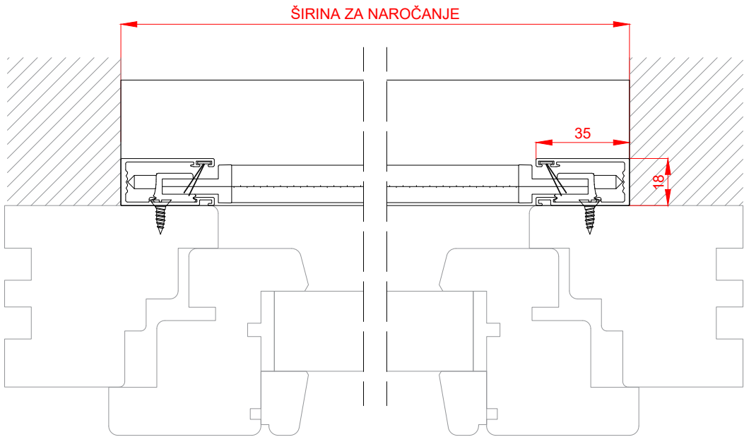
Horizontalni prerez:
