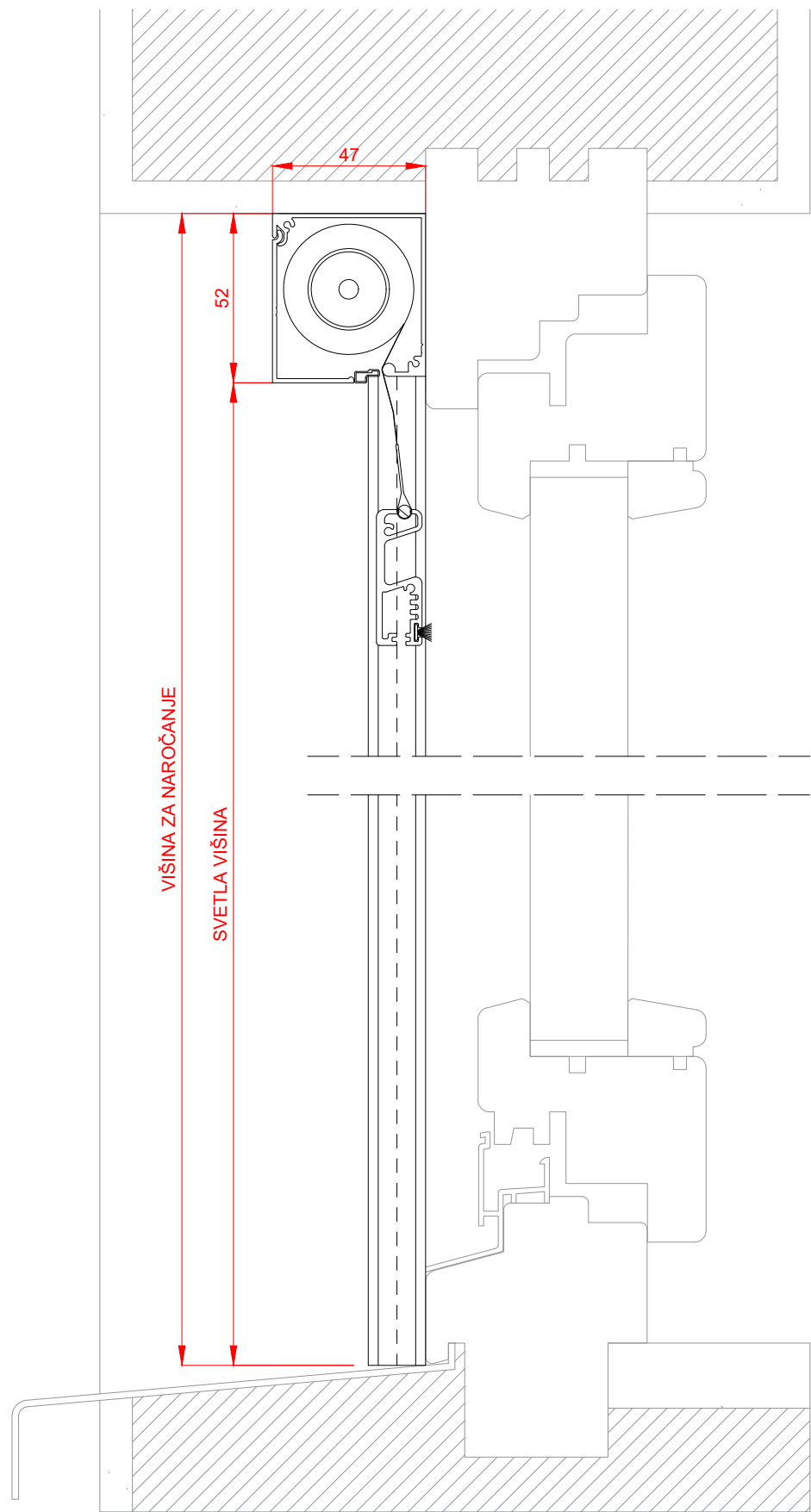
Vertikalni prerez:
