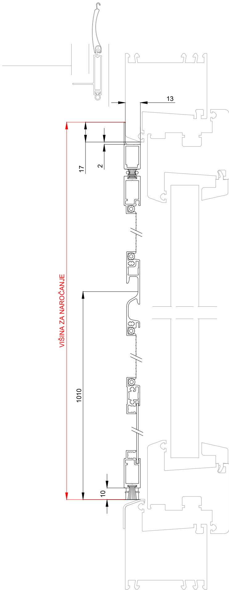
Vertikalni prerez:
