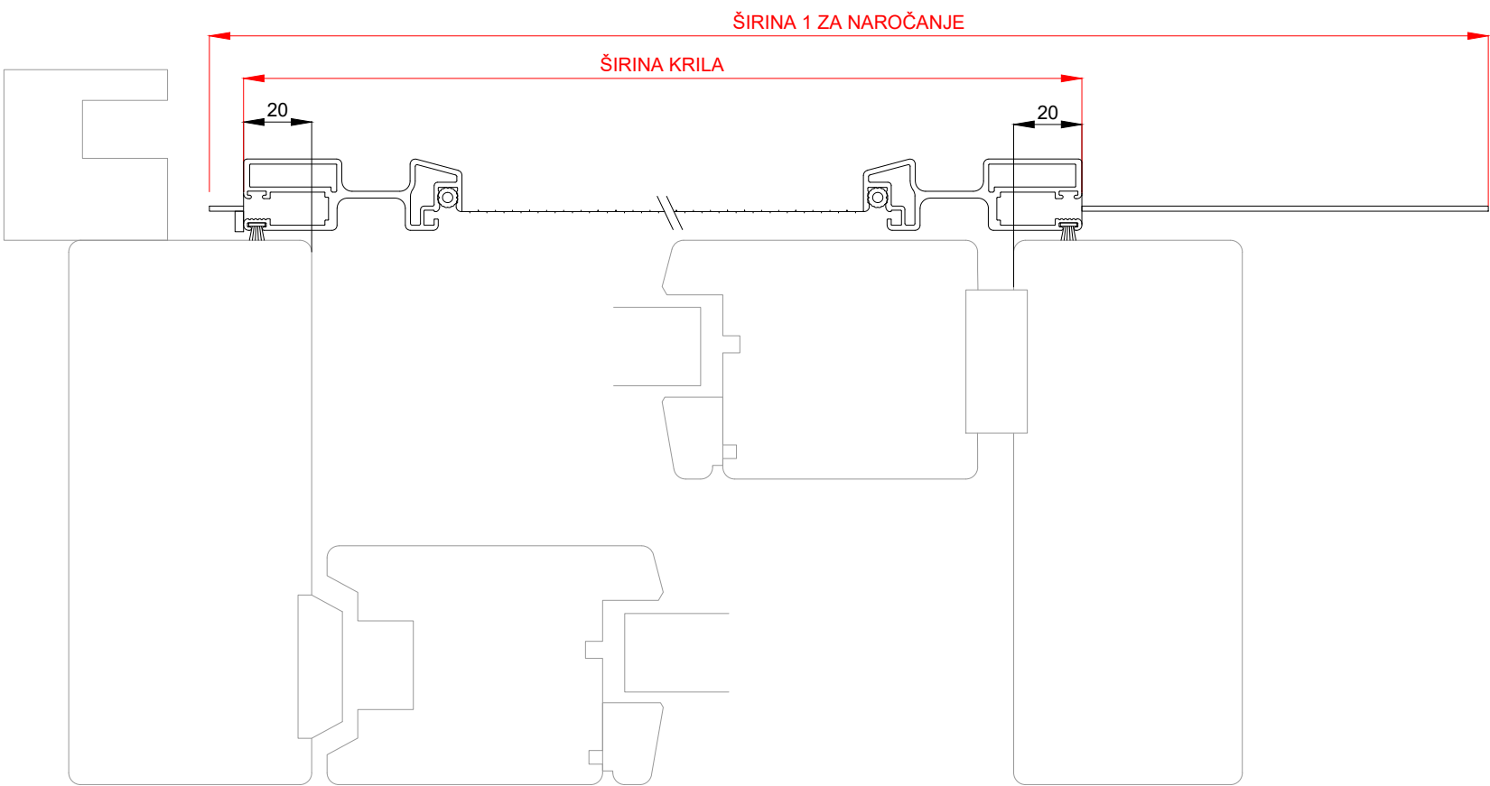
Horizontalni prerez:
