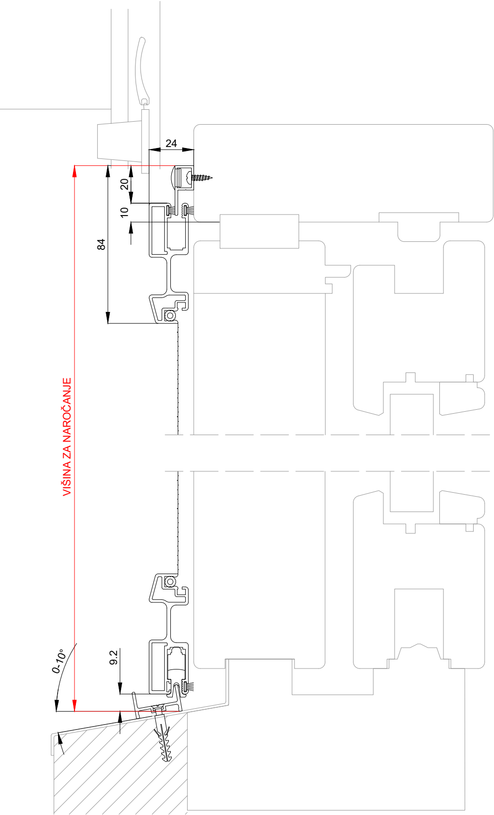
Vertikalni prerez:
