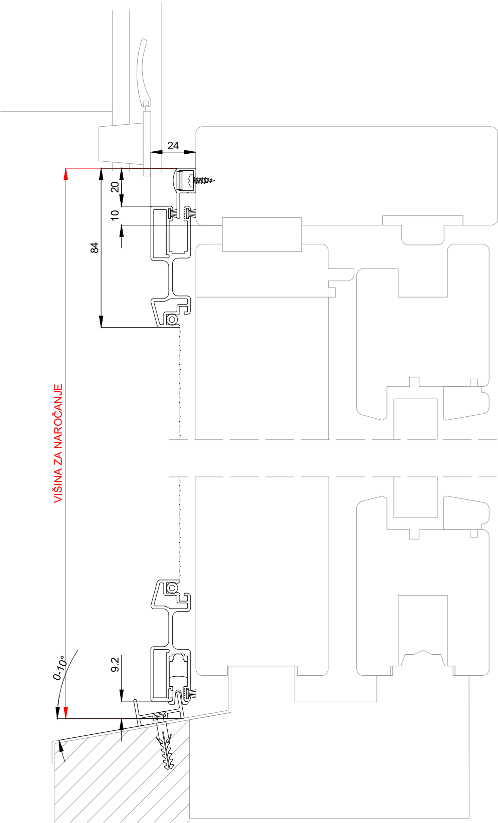
Vertikalni prerez:
