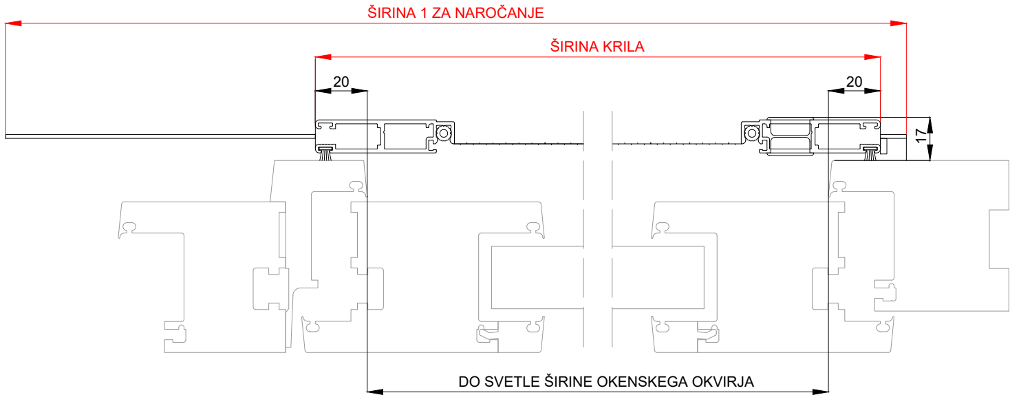
Horizontalni prerez:
