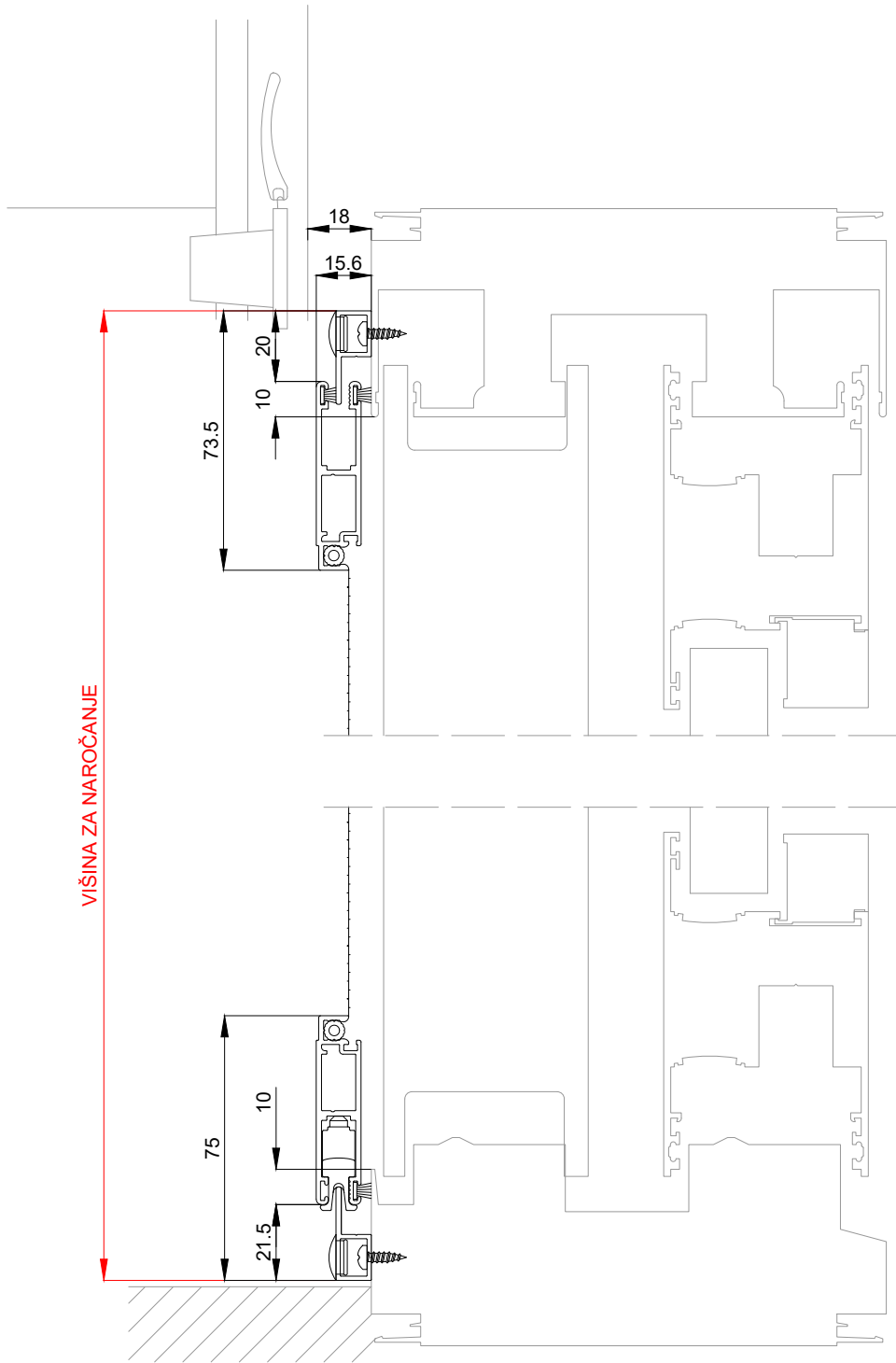
Vertikalni prerez:
