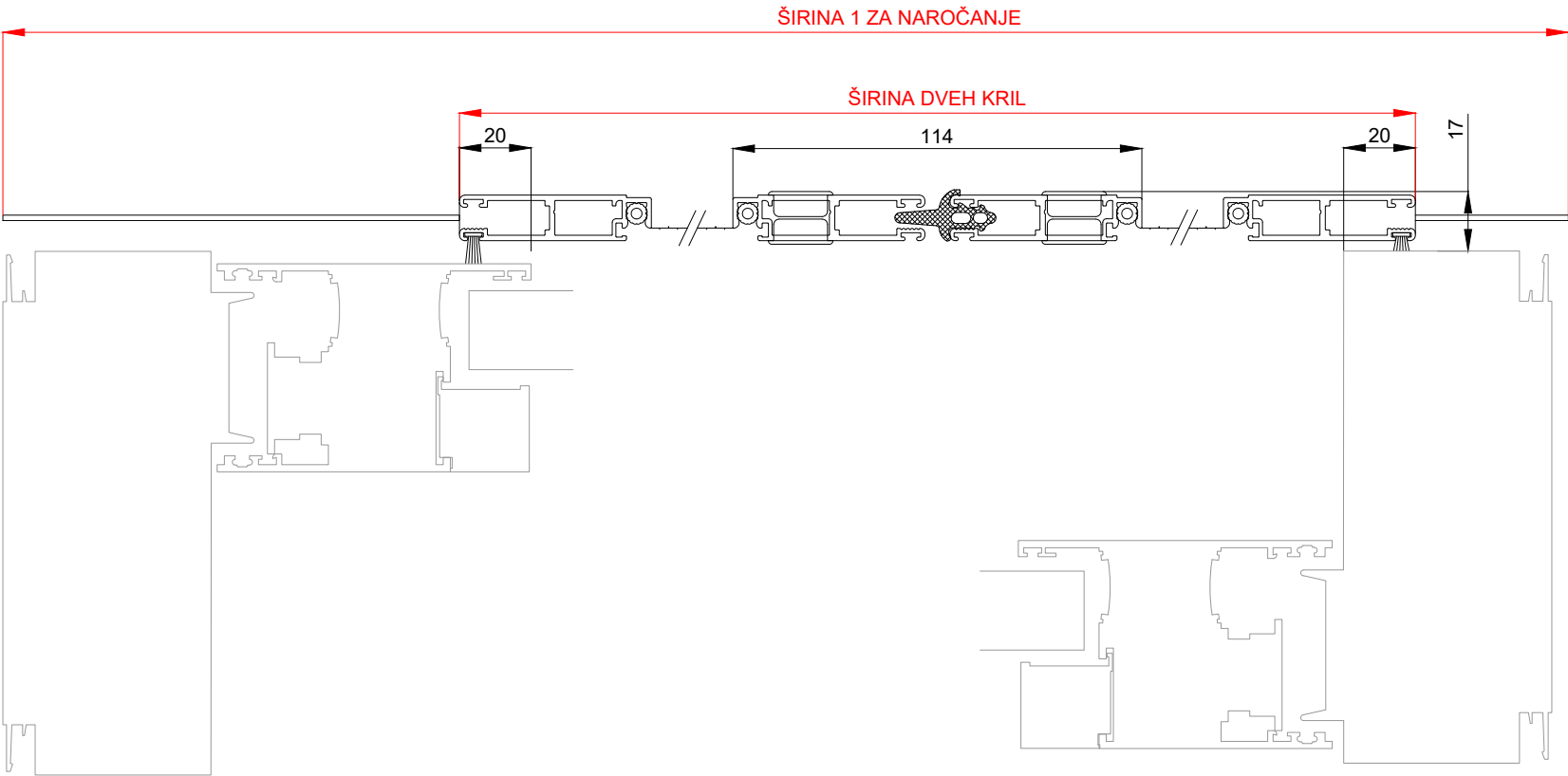
Horizontalni prerez:
