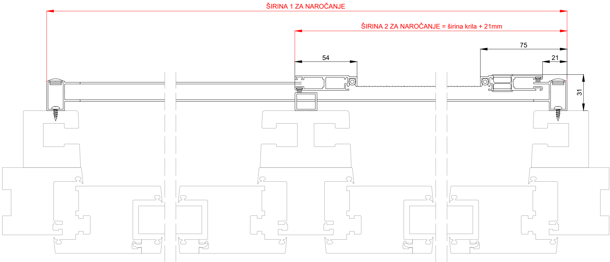
Horizontalni prerez:
