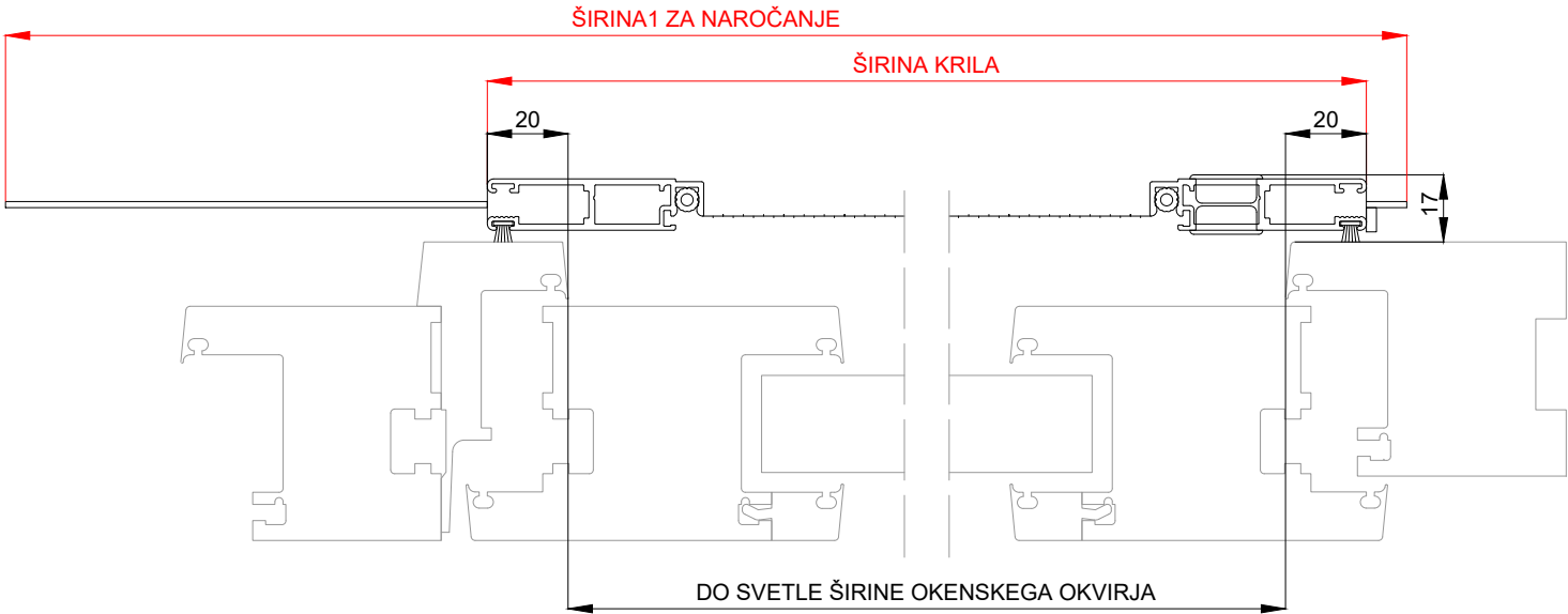
Horizontalni prerez:
