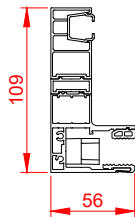
Führungsschienen mit Glasabsturzsicherung
