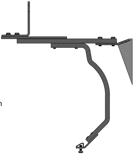
Blendrahmenstabilisierung EB > 2000 mm
