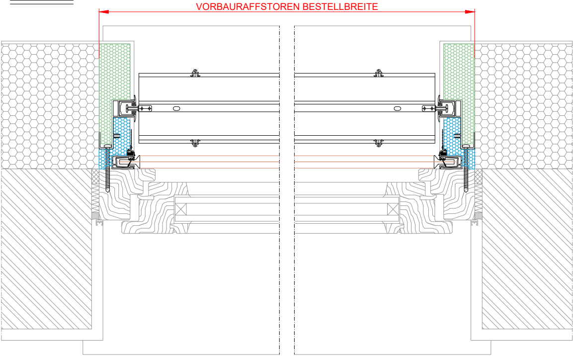
Schnitt 1-1
