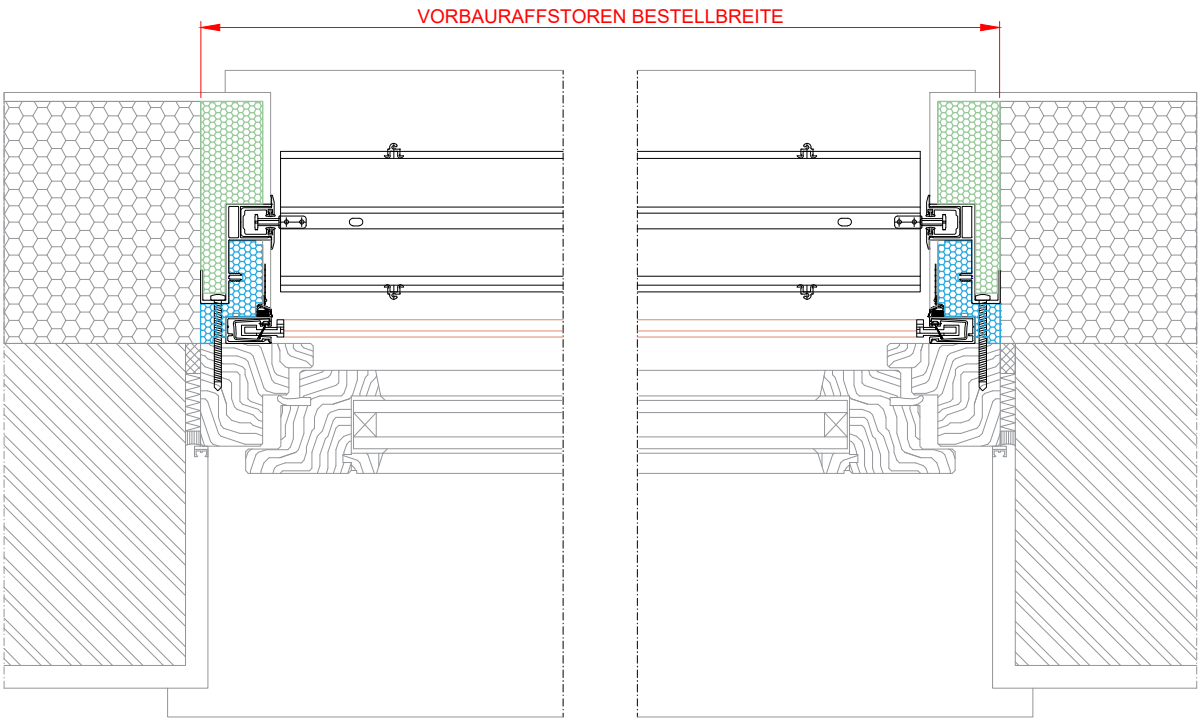
Schnitt 1-1
