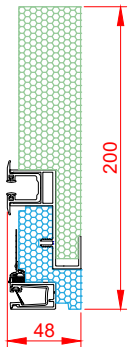
Führungsschienen
