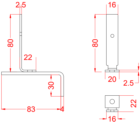
Enojni talni odmični nosilec vodil HERO.2
