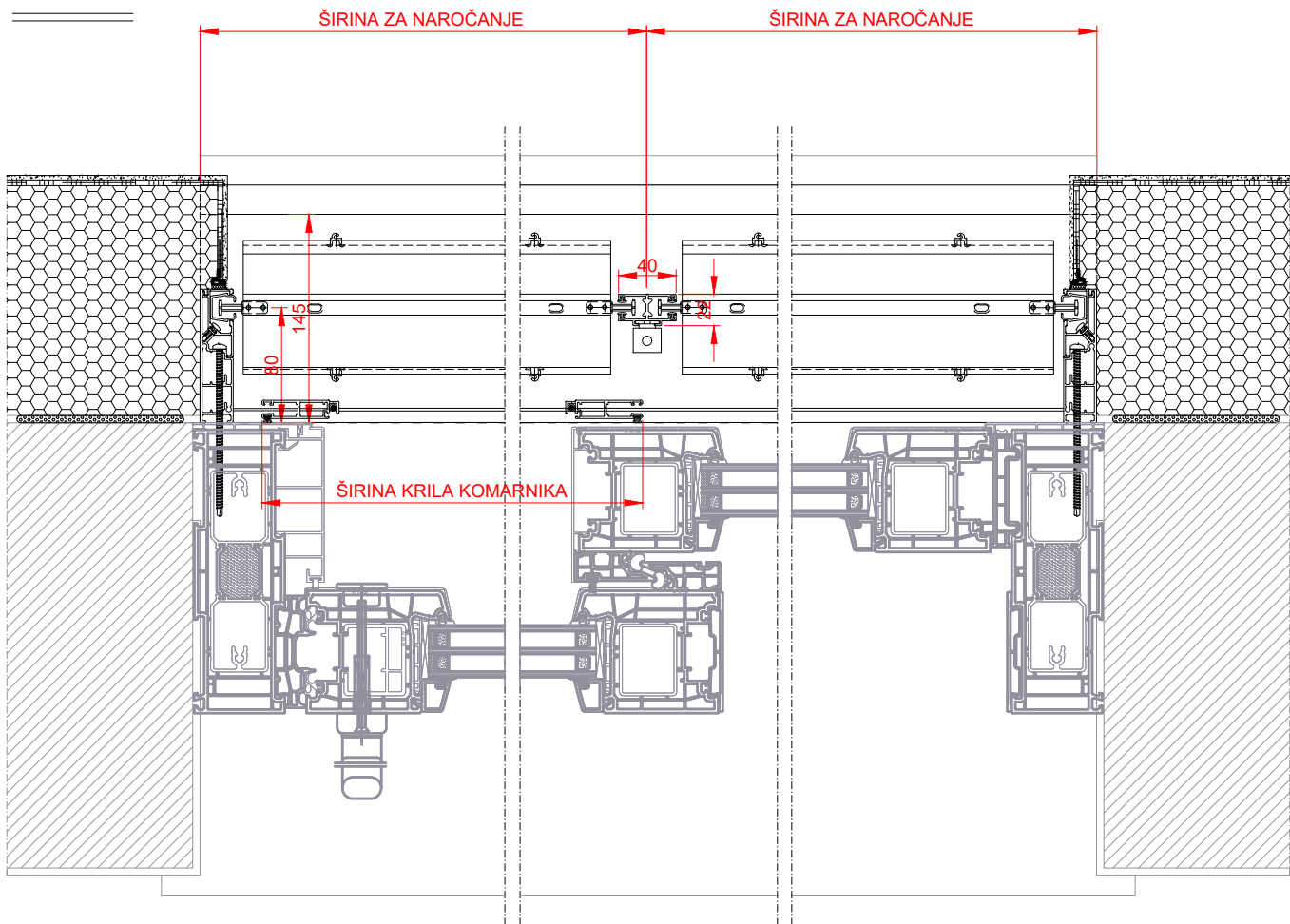
Prerez 1-1
