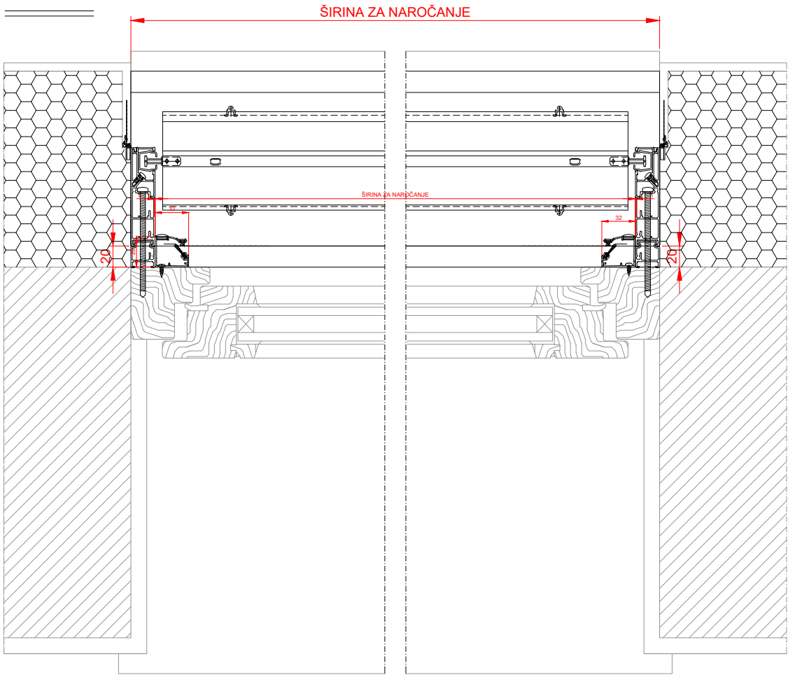
Prerez 1-1
