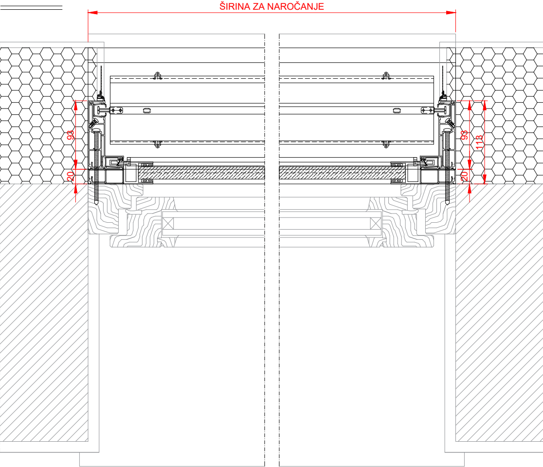
Prerez 1-1
