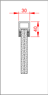
Stirodur 20 mm
