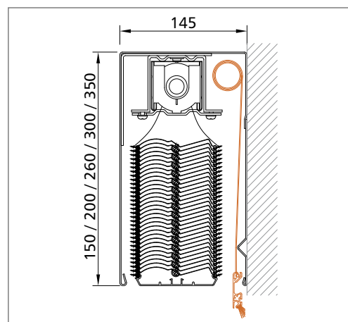
HERO.1X sistem, vidna izvedba
