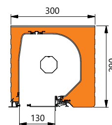
omarica z žaluzijami
