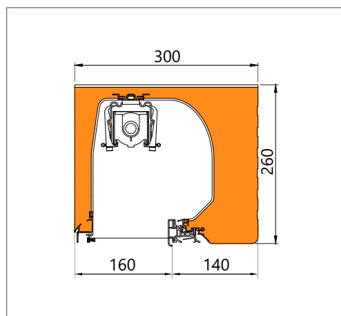
HERO.5 sistem, podometna izvedba
