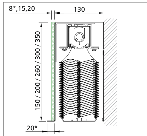
HERO.1 sistem, podometna izvedba
