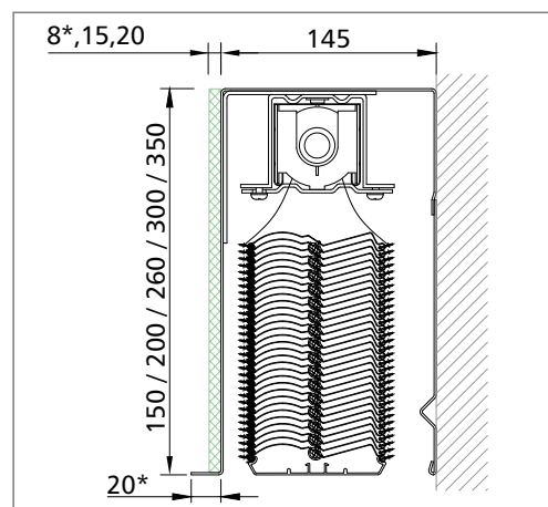
HERO.3 sistem, podometna izvedba
