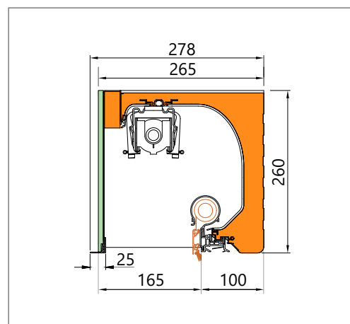
HERO.5X sistem, podometna izvedba
