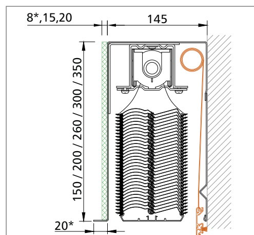
HERO.3X sistem, podometna izvedba
