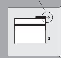
Primer: krmiljenje enega pogona z enim stikalom.
